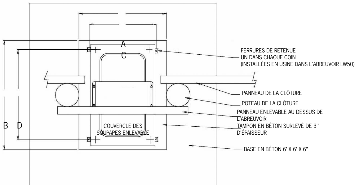
DIAGRAMME 1 - EMPLACEMENT ET MONTAGE DE L'ABREUVOIR (VUE DU HAUT D'UN ABREUVOIR INSTALLÉ LE LONG D'UNE CLÔTURE)
